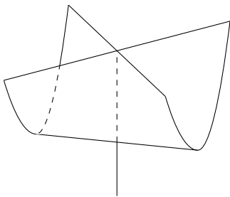
图 2.1. Whitney 伞 X^2 - Y^2Z = 0 的实数部分
