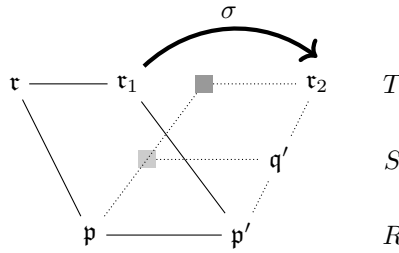
图 6.1. 定理 6.6.3 (v) 的论证示意
