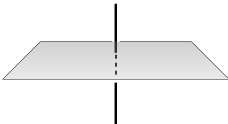
图 8.1. 对应 \mathbb{k}[X, Y, Z]/(XZ, YZ) 的几何图像
