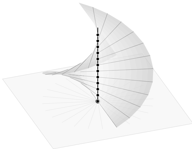
图 4.1. 对于例 4.6.5 的直观图像
